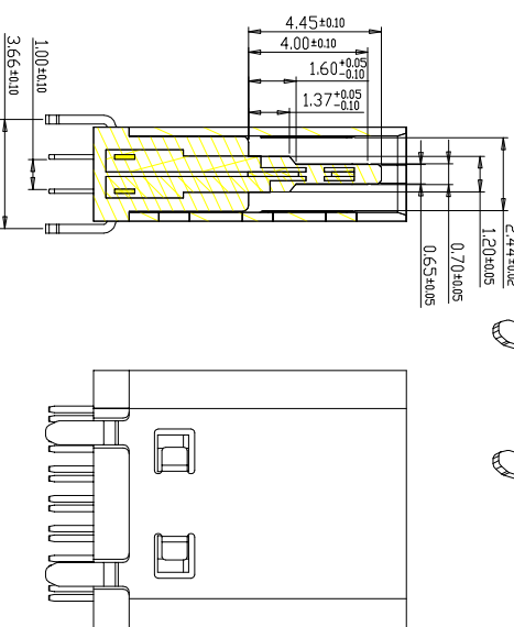
1-1 截面
