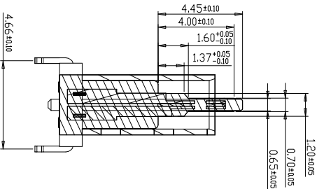
截面 1-1
