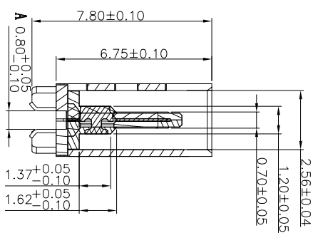
截面 A-A
