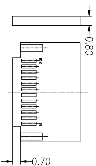
PCB 板焊点示意图
