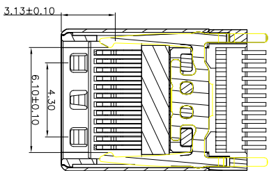
截面 D-D
