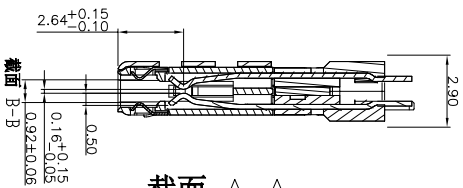
截面 A-A
