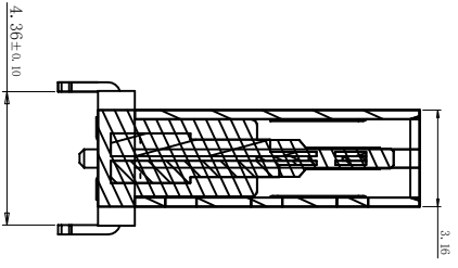
截面 1-1
