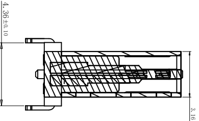
截面 1-1
