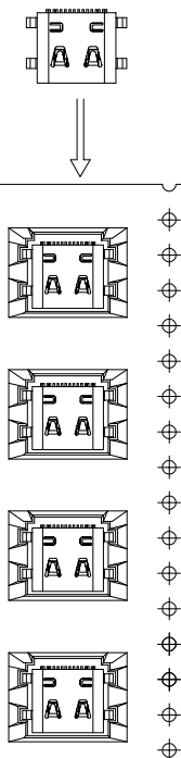
② 产品入载带示意图
