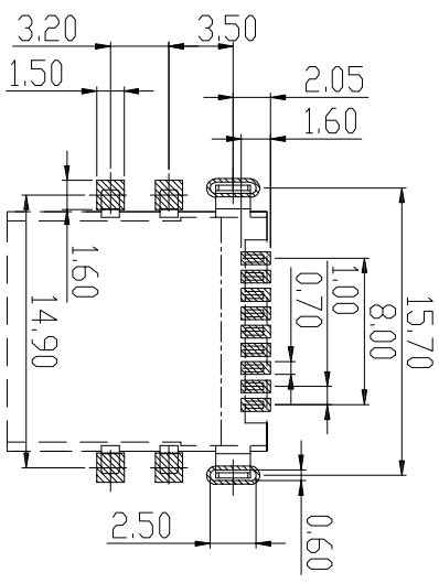
参考 PCB
