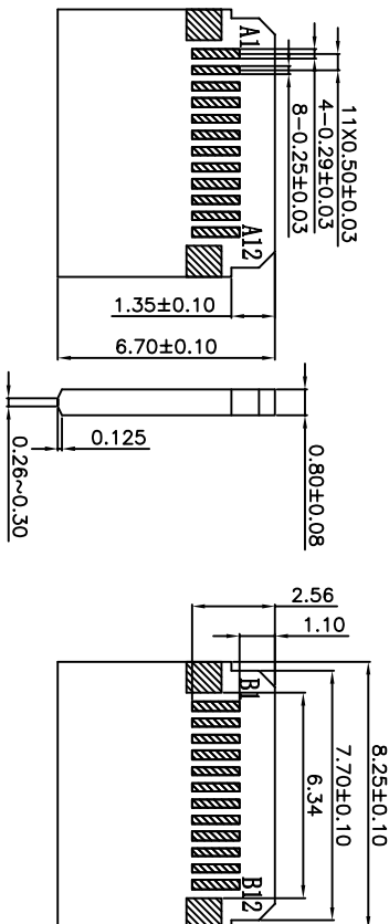
pch layout参考图
