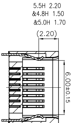
SECTION D-D
