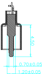
SECTION A-A SCALE 1:1
