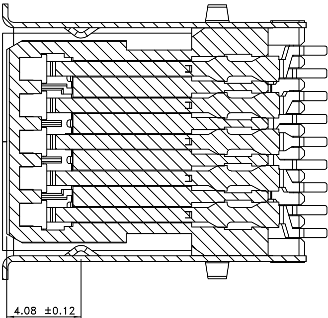
剖面圖 B-B
