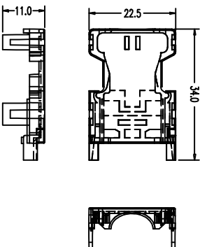
上壳
