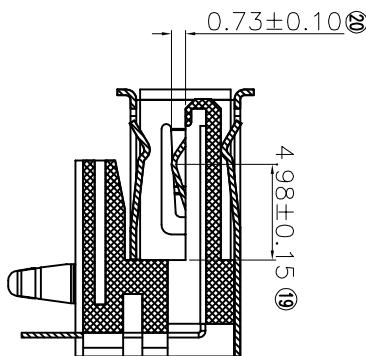
截面B-B
