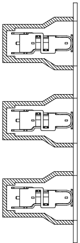
① 产品入载带示意图
